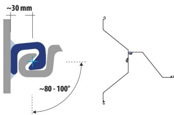
Вариант соединения Z-образных шпунтовых свай
