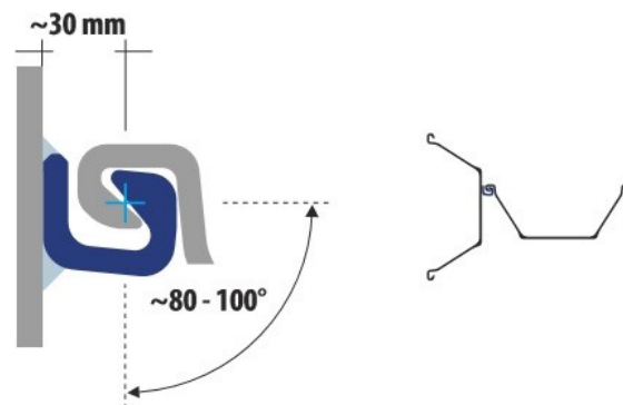
Вариант соединения U-образных шпунтовых свай
