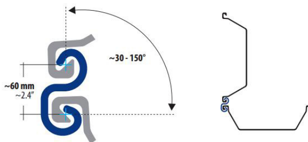
Вариант соединения U-образных шпунтовых свай
