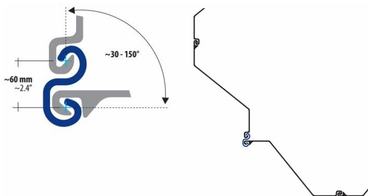
Вариант соединения Z-образных шпунтовых свай
